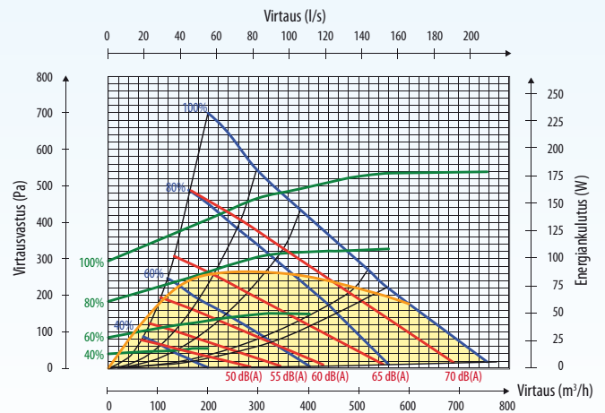
Poistoilman puoli (F7 suodattimella)
