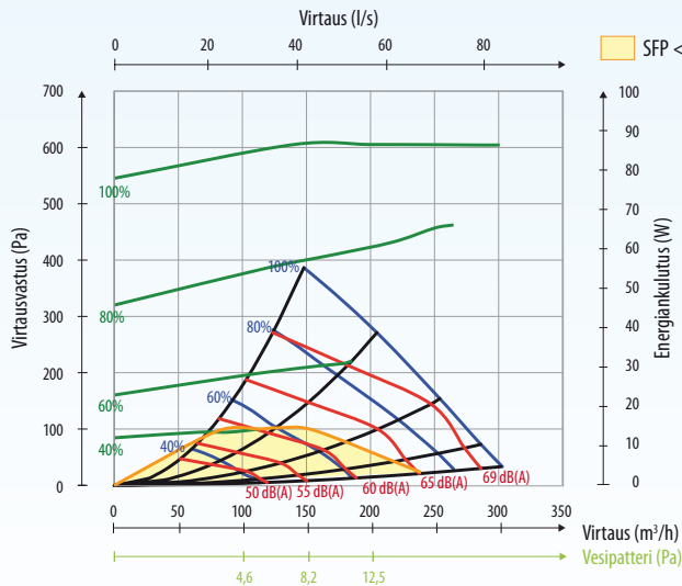
Tuloilman puoli (F7 suodattimella)
