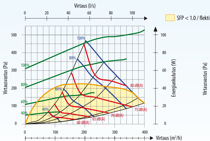
Tuloilman puoli (F7 suodattimella)
