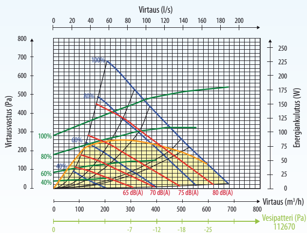
Tuloilman puoli (F7 suodattimella)
