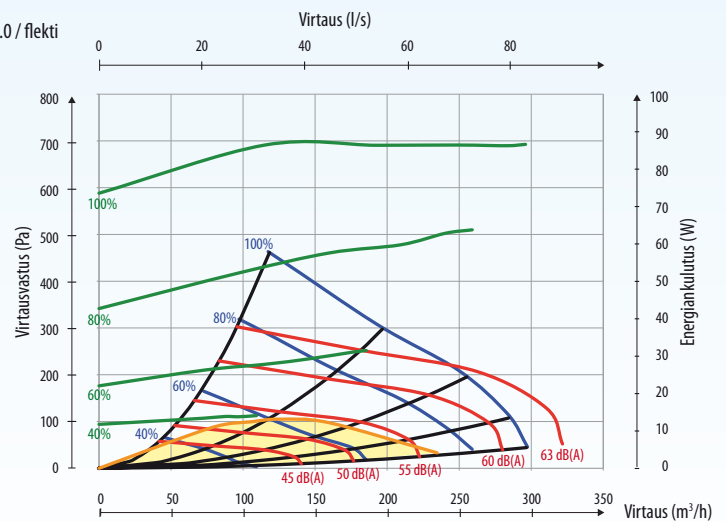
Poistoilman puoli (F7 suodattimella)
